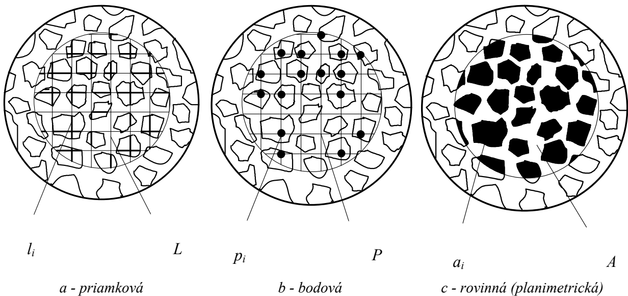
Obr. 5. Metódy hodnotenia objemového podielu skúmanej fázy
