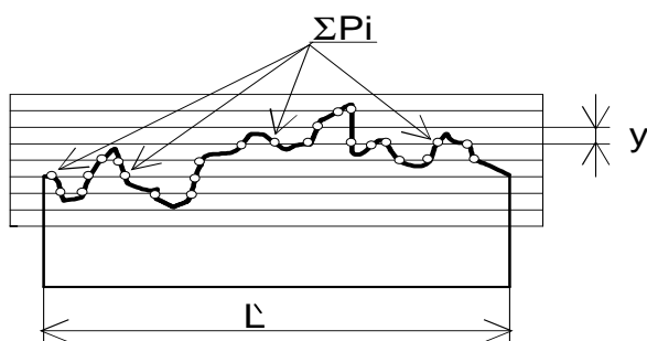
Obr.1 Postup určenia súčiniteľa R_v metódou priesečníkov profilovej krivky lomu s testovacou mriežkou
