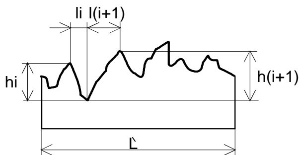
Obr.2 Postup určenia súčiniteľa R_v metódou merania rozmerov a vzdialeností vyvýšení a priehlbín
